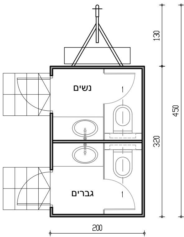
תכנית קרון ריף
